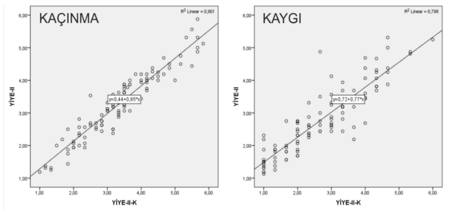
Şekil 1: YİYE-II-K Ölçeği ile YİYE-II Ölçeğinin Boyutlar Bazında İlişisini Gösteren Serpm Diyagram
