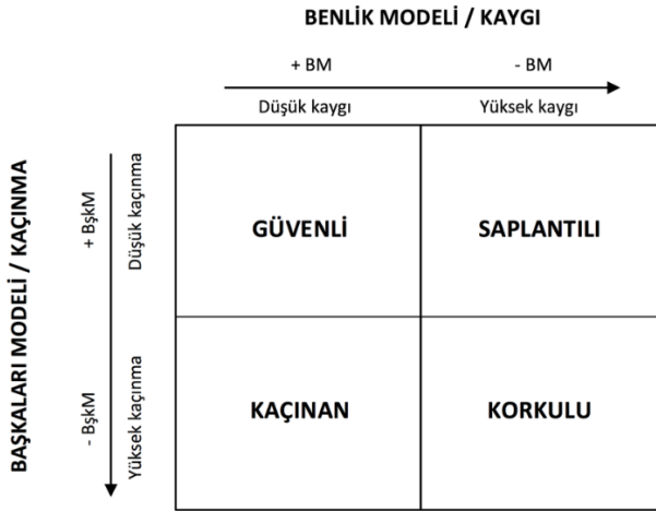
Şekil-1: Dört Kategori Modeli
