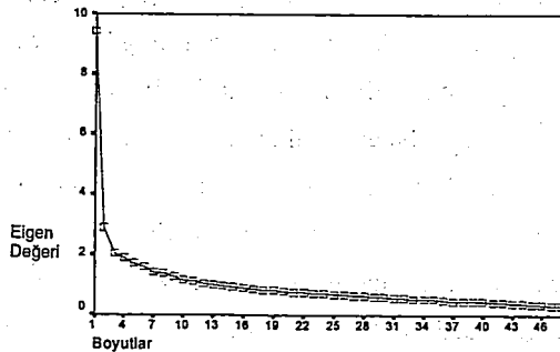
Şekil 1: Scree Test
