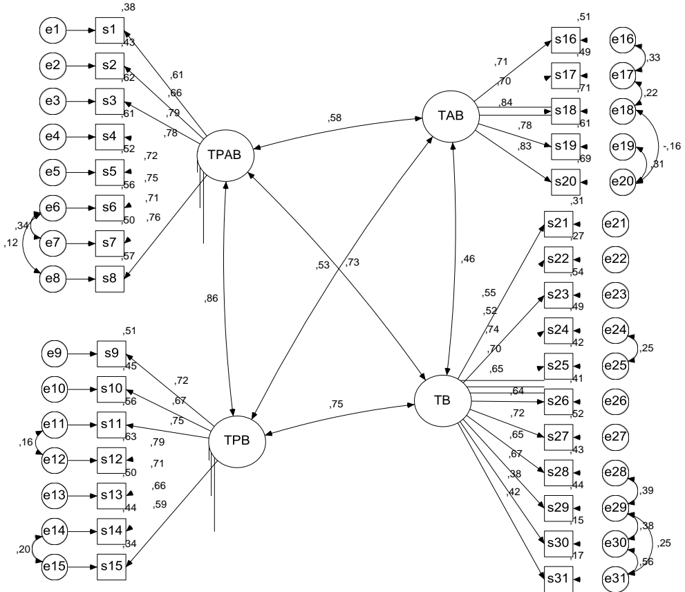
Şekil 3. İkinci DFA
