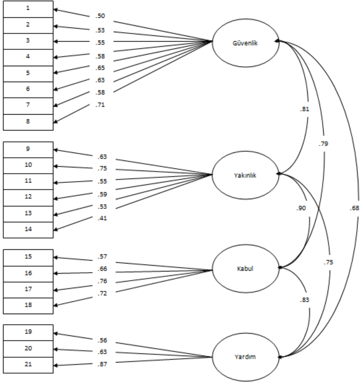
Şekil 1: Arkadaşlık Kalitesi Ölçeği'ne İlişkin Path Diagramı ve Faktör Yükleri
